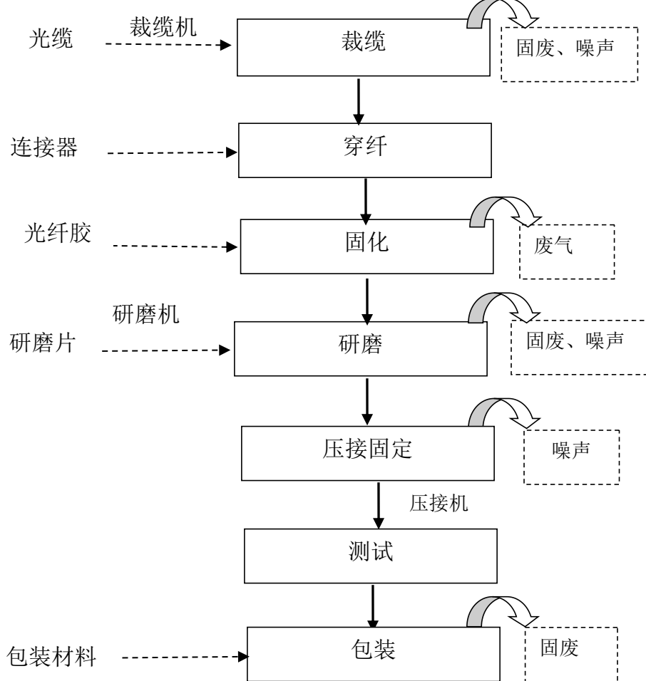
图-1 生产工艺流程及产污过程图
